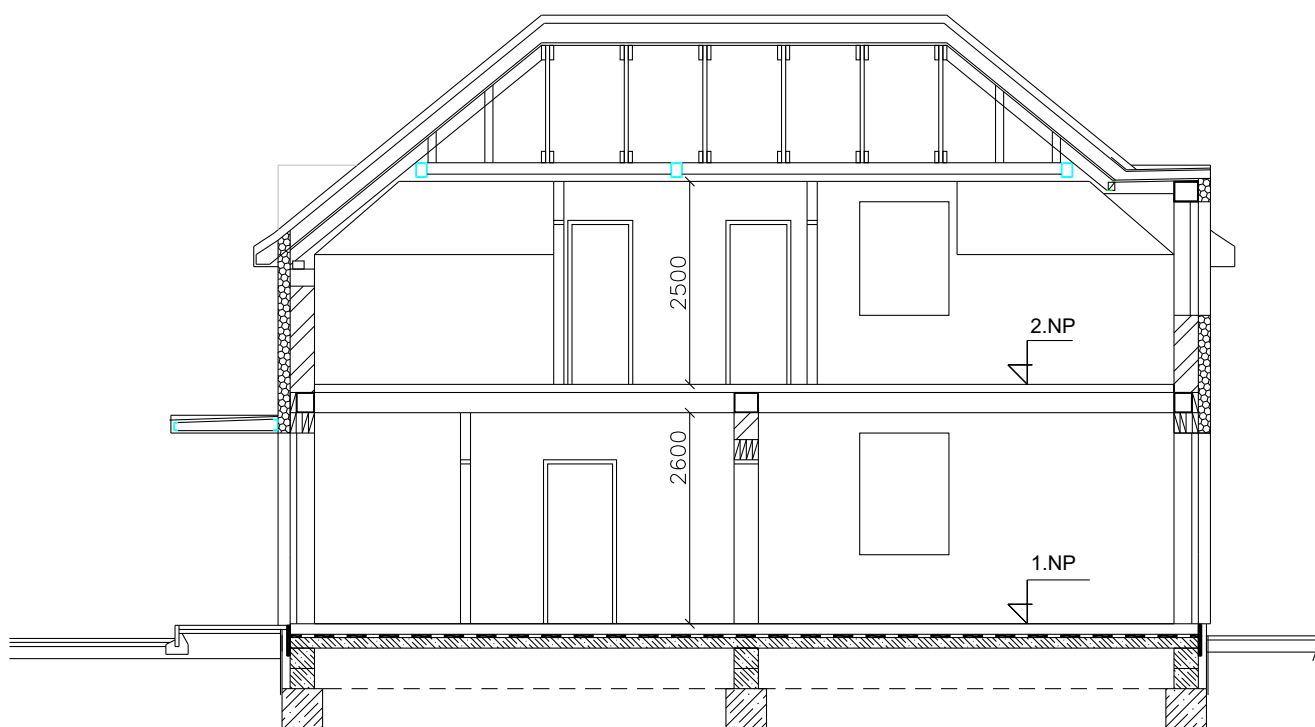
ŘEZ DOMU
