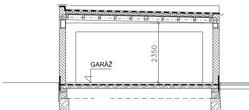
ŘEZ GARAŽE
