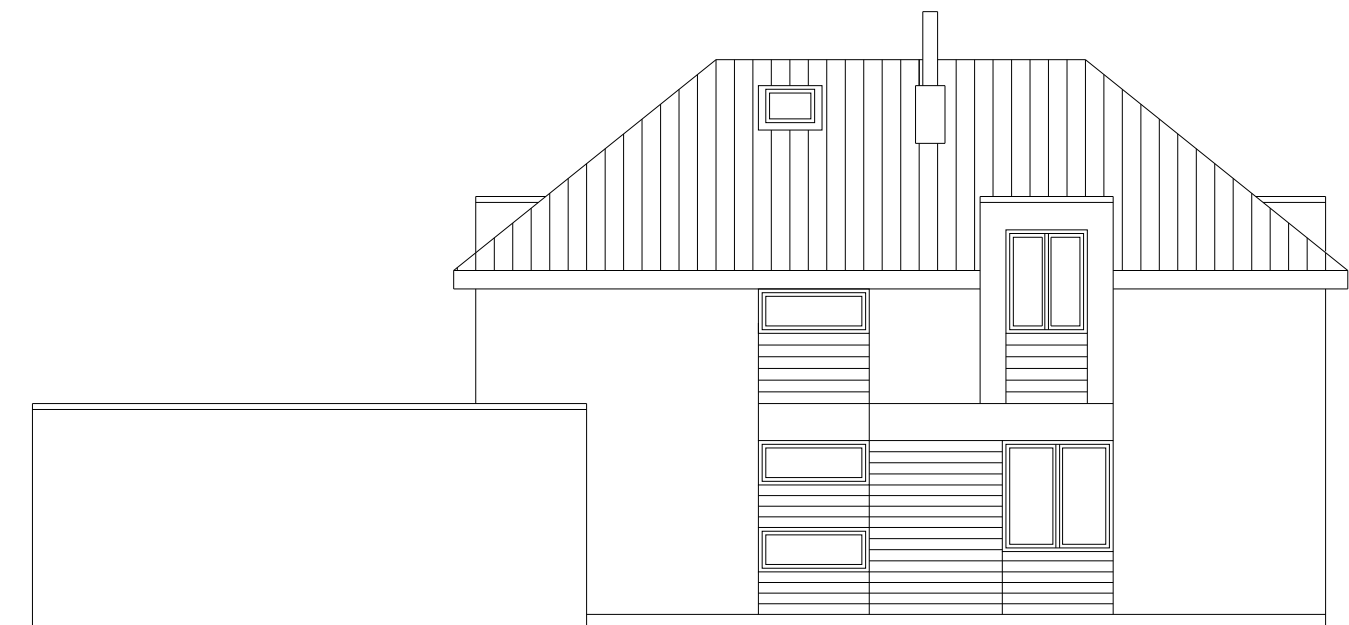
Pohled boční - severní
