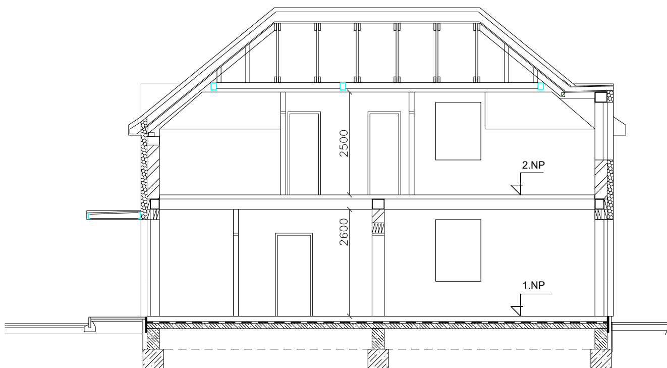
ŘEZ DOMU
