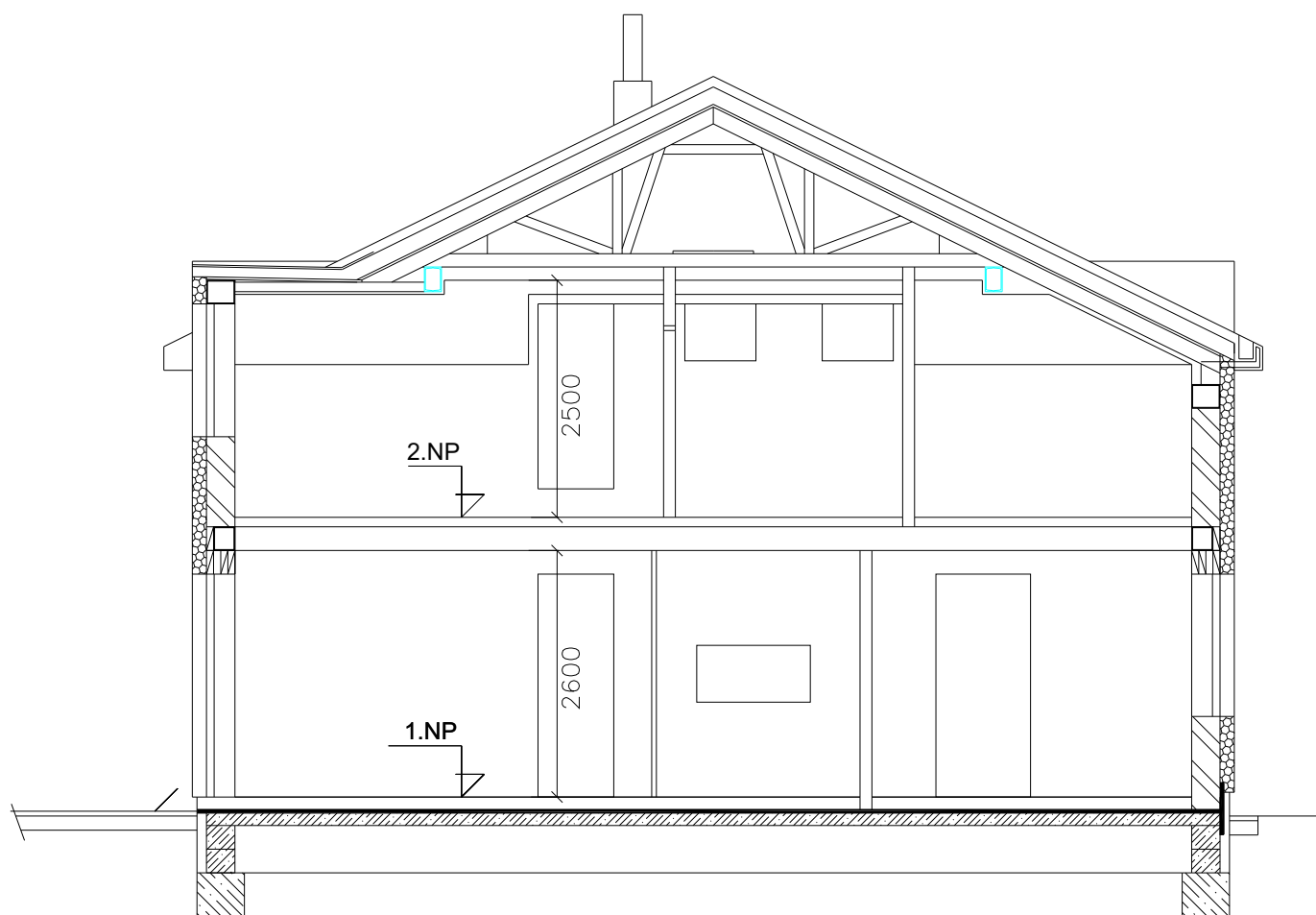
ŘEZ DOMU
