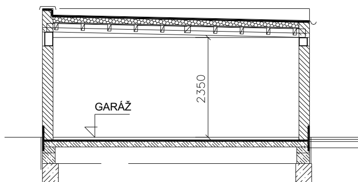
ŘEZ GARAŽ
