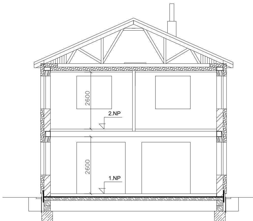
ŘEZ RD
