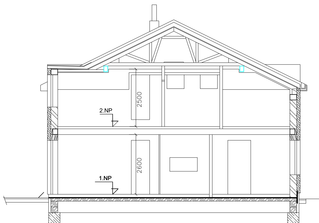
ŘEZ DOMU
