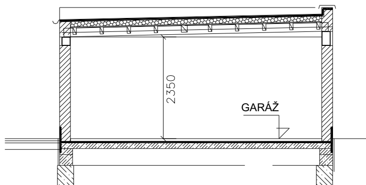
ŘEZ GARAŽ
