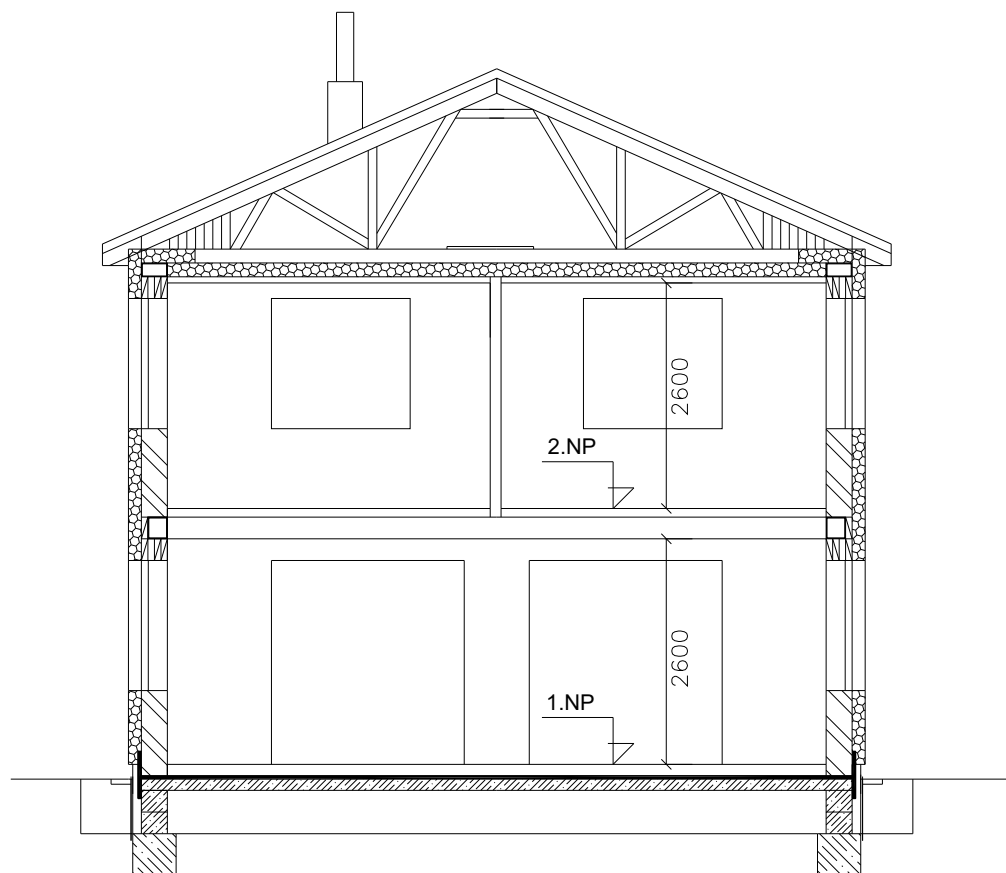
ŘEZ RD
