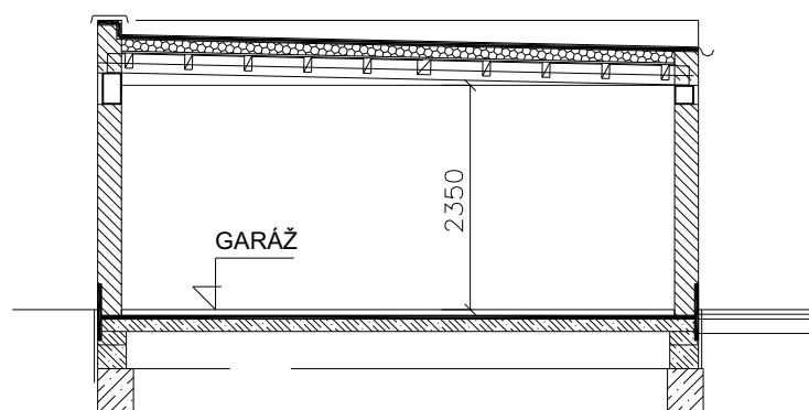
ŘEZ GARAŽ
