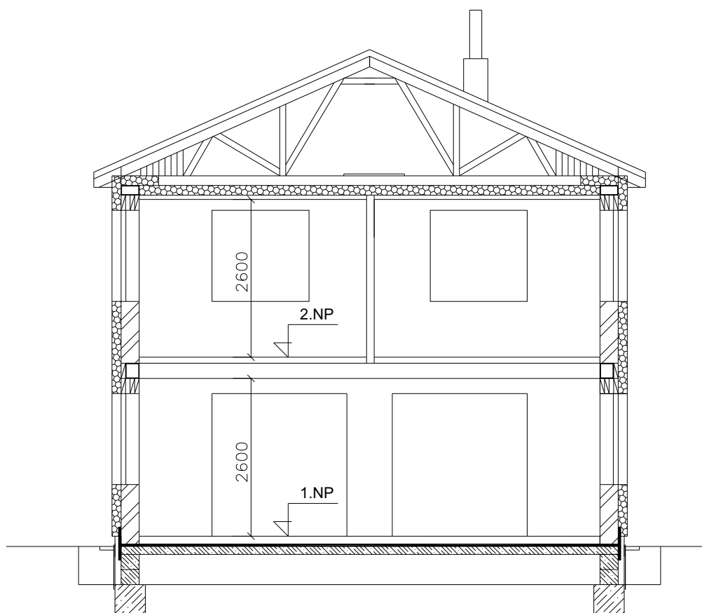
ŘEZ RD
