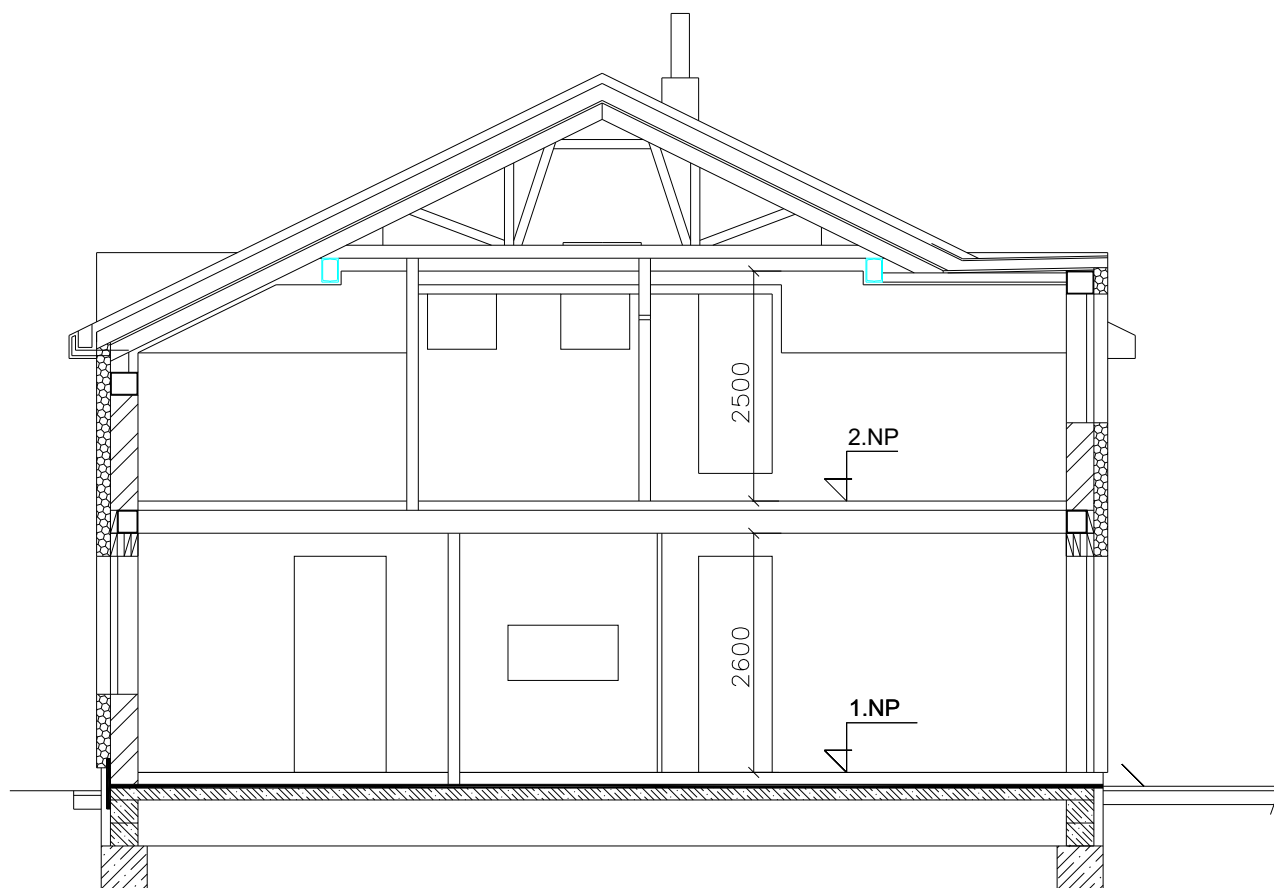
ŘEZ DOMU
