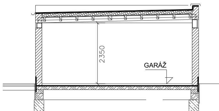
ŘEZ GARAŽ
