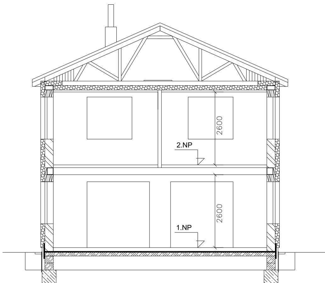
ŘEZ RD
