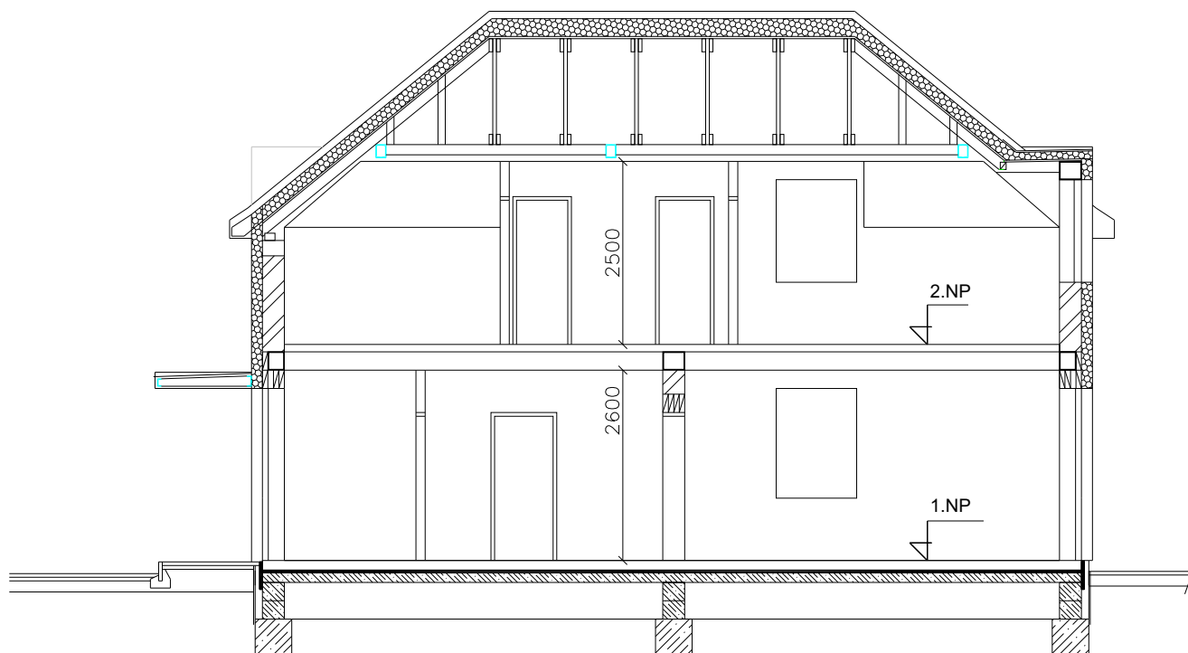
ŘEZ DOMU
