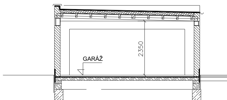
ŘEZ GARAŽE
